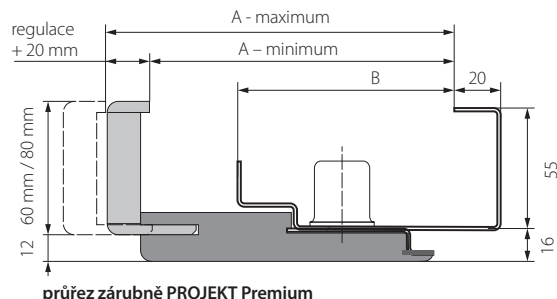
průřez zárubně PROJEKT Premium
