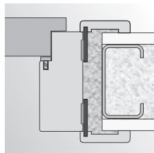
montáž na pěnu do stěny SDK
